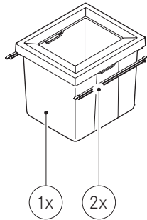
FX 45 35 (FUN 121.0557.744)
